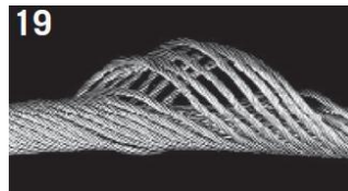
19 Vznik košíku na nekroutivém ocelovém laně. Pokud je vidět jedno, jsou vidět všechny.
